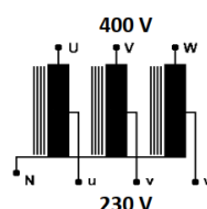
Fig.2: electrisch schema
